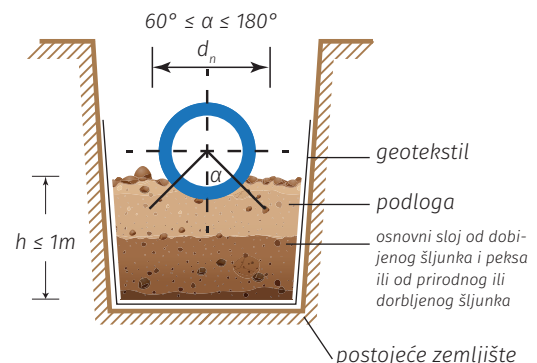
Primer polaganja na slabo nosivom tlu debljine ≤1.0m
