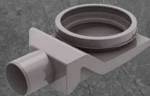
Ultra niska S baza sa 25 mm vodenim čepom
