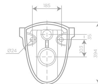
BASIC WC ŠOLJA SA CLICK DASKOM
