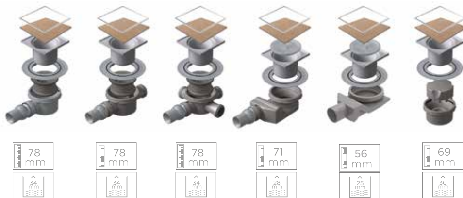
Modeli sa 10x10 rešetkom
