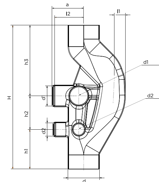
POGLED NA PRESEK ODNOS: 1:5
