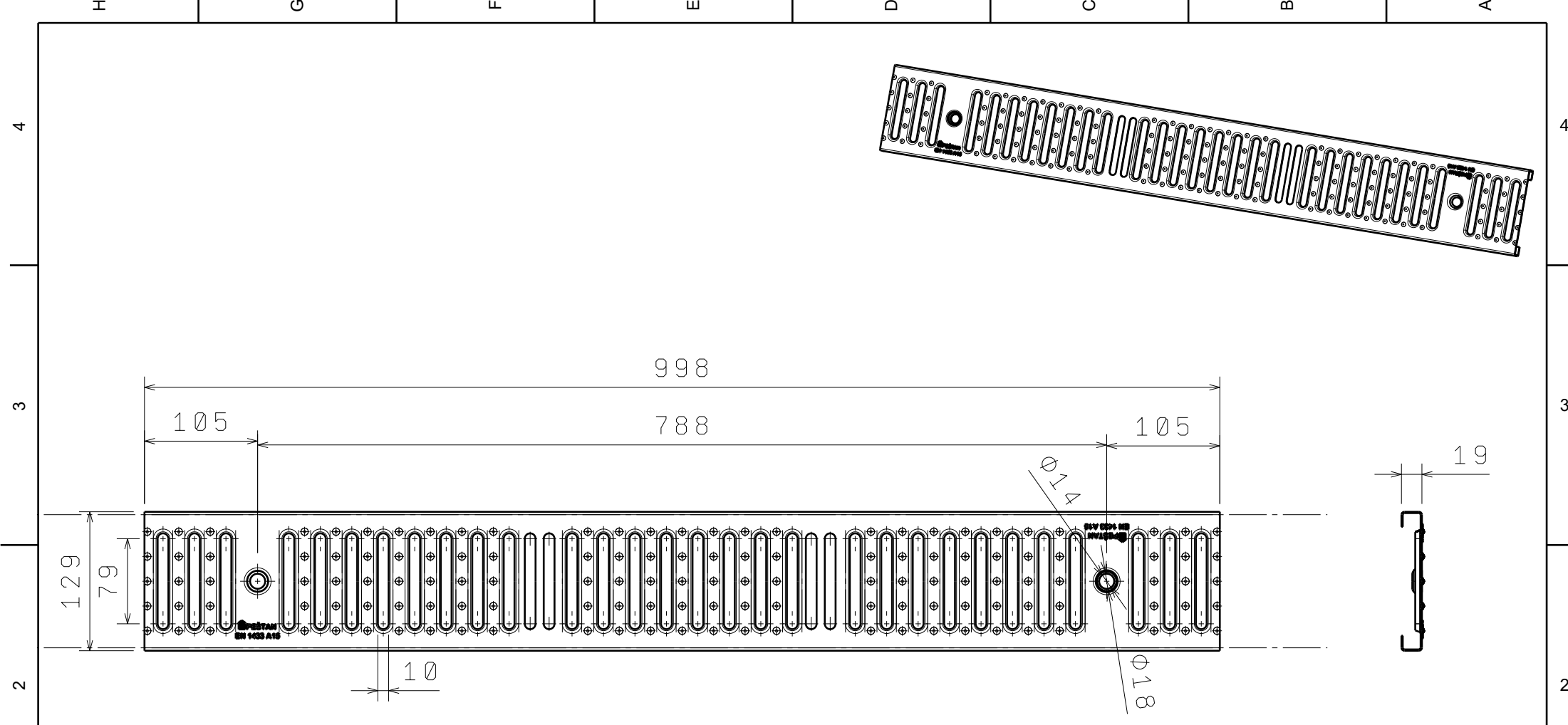
Left view Scale: 1:5
