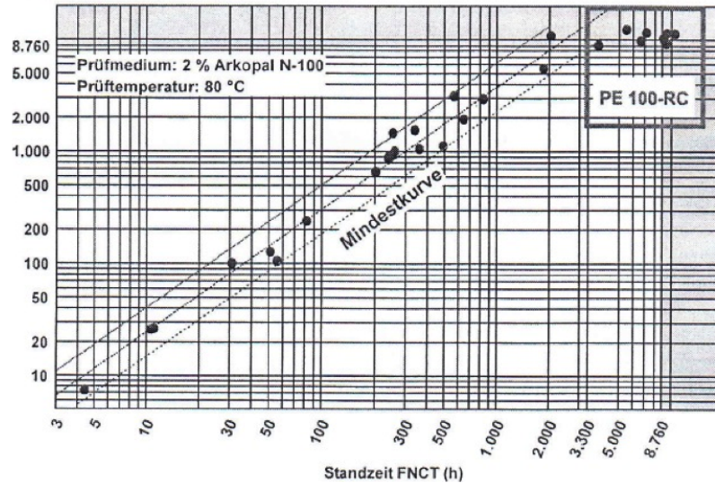
Standzeit Rohr mit Punktlast (h)
