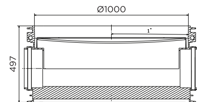
Inlet/outlet DN250
