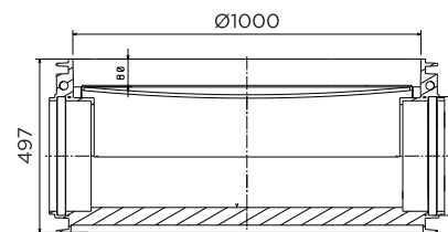
Inlet/outlet DN315
