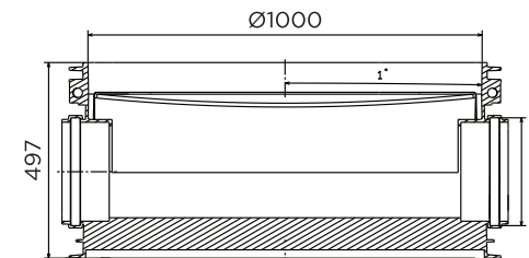
Ulaz/izlaz DN250
