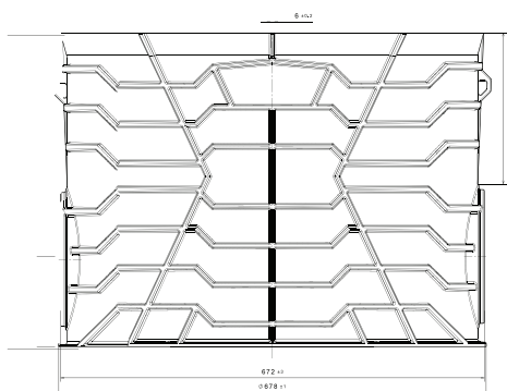
Tehnički crtež slivničko dno prolazno 630/200
